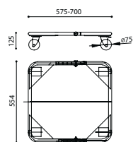
STACCATO WAGEN STACCATO CART
