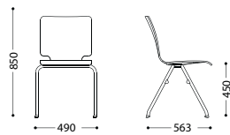
AXO 2
