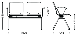
AXO 3
