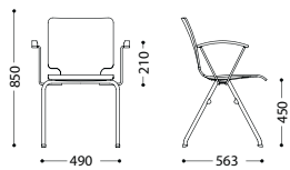
AXO 1
