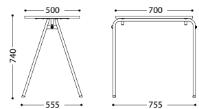
AXO TABLE
