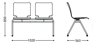
AXO 4
