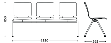
AXO 6
