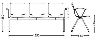
AXO5
